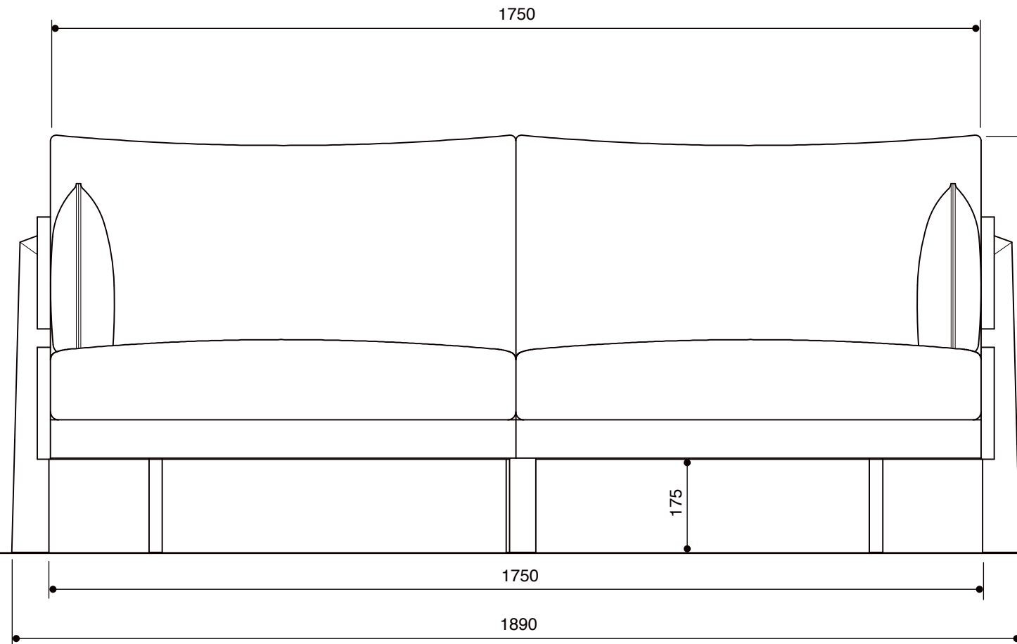
【正面】
