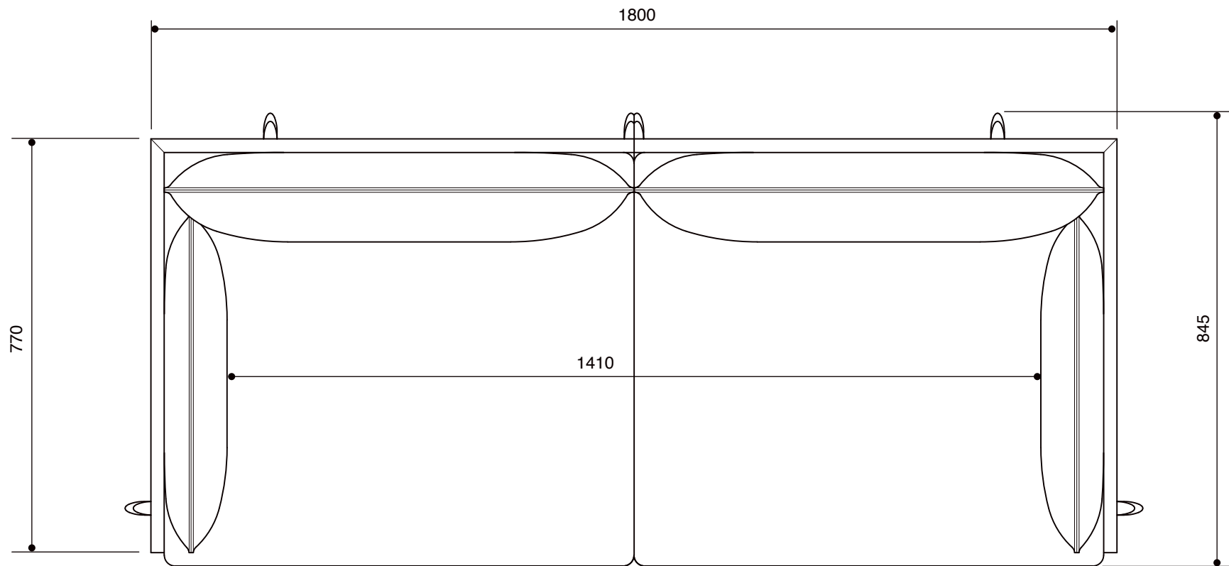
【平面】
